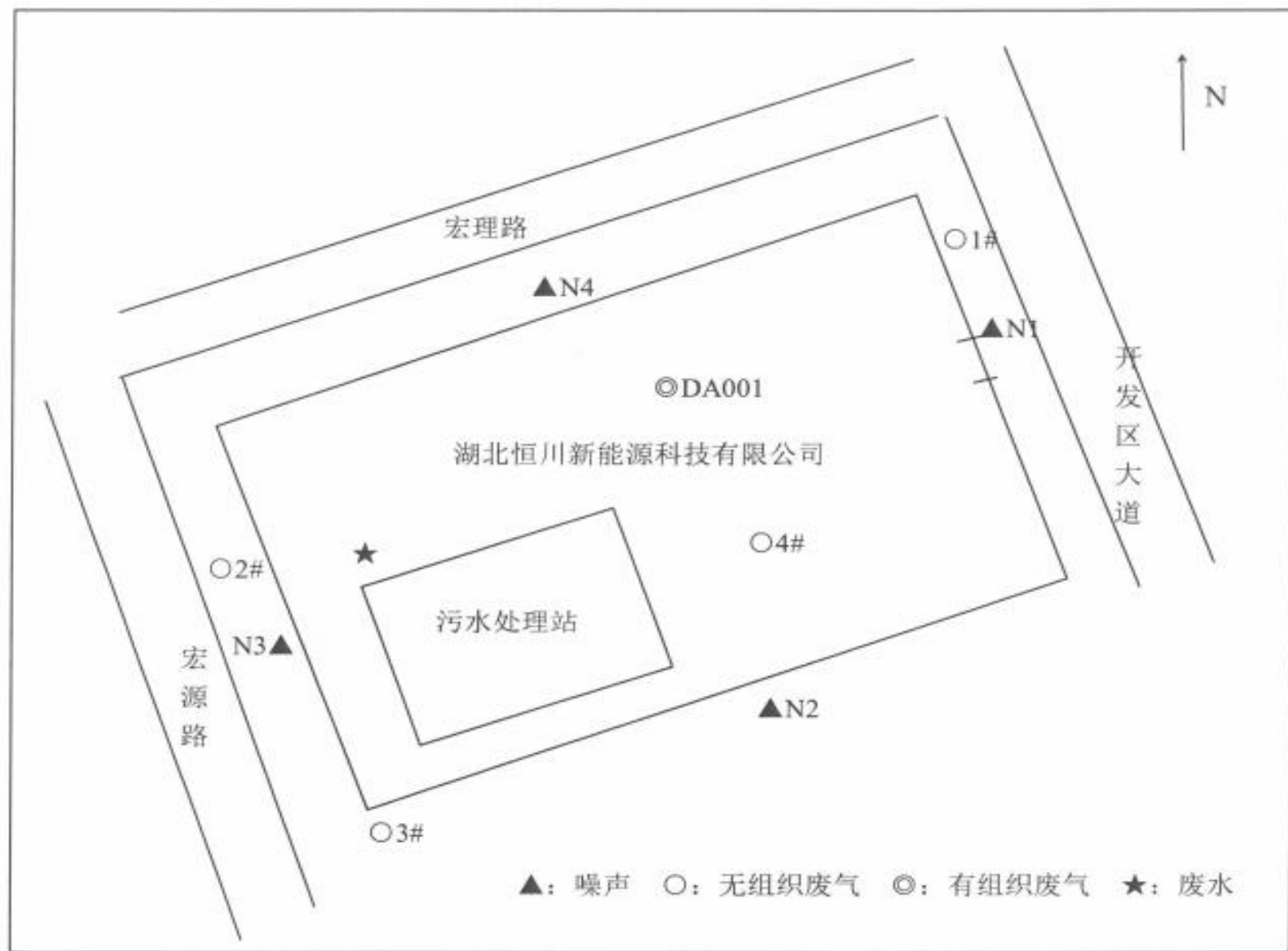
附图5 验收监测点位图
