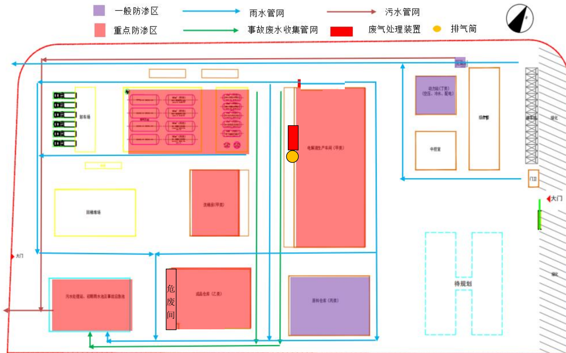
附图 4 项目分区防渗图 (含雨污管网图)
