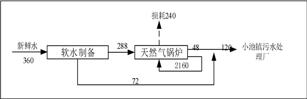
图 2-2 项目水平衡图（单位：t/a）
