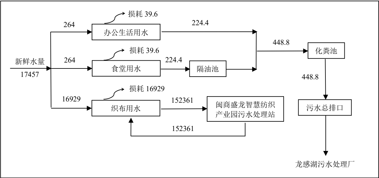
图 2-2 项目水平衡图（单位：m³/a）
