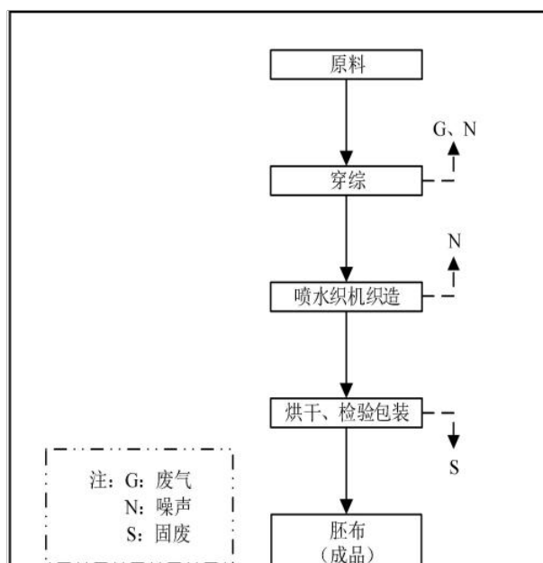
图 2-3 生产工艺流程及产污节点图
